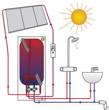
Solar 300 нагревает ГВС с помощью солнечной энергии.
