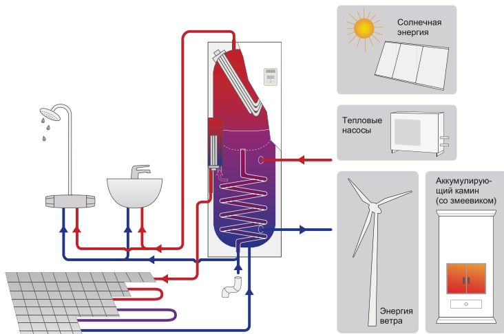
Ecowatti можно подключить к нескольким источникам возобновляемой энергии.
