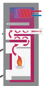
Пеллетный котел Pelletti 20 в поперечном разрезе
