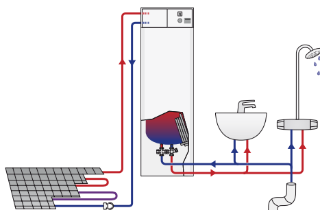
Электрокотел Pikkuwatti можно монтировать параллельно с водонагревателем VLM.
