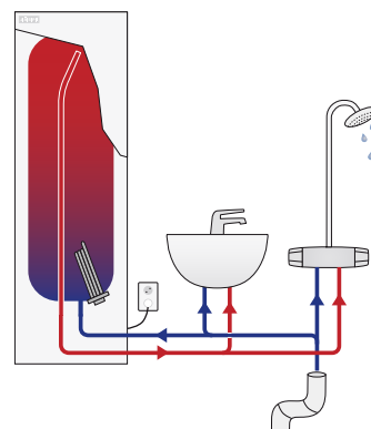
VLM нагревает ГВС.
