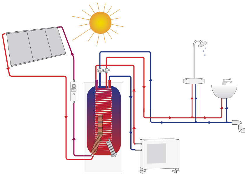
VLM 300 KS Star подключенный к тепловому насосу и солнечным панелям
