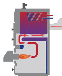
Дизельная / газовая топка Biotriplex
