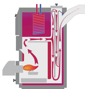
Пеллетный котел Pelletti XL в поперечном разрезе
