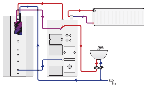
Подключение Tupla к аккумулятору энергии GTV.
