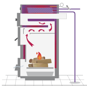
Дровяной котел YPV в поперечном разрезе
