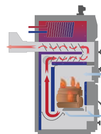
Дровяная топка Biotriplex
