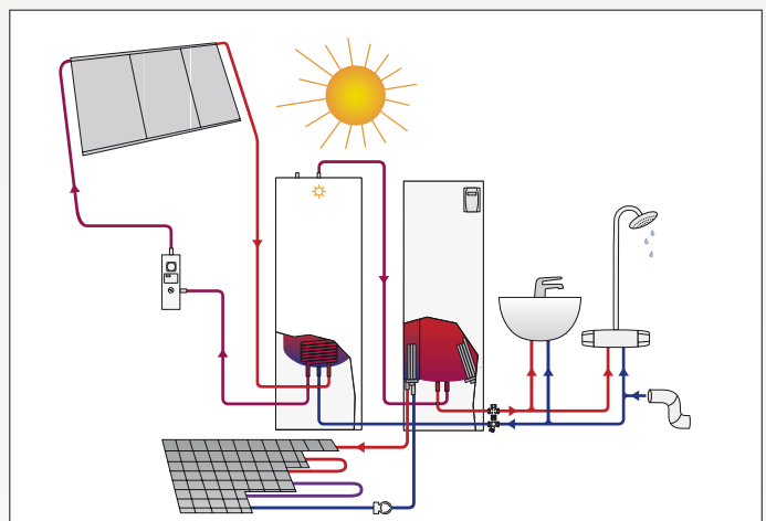
Подключение аккумулятора солнечной энергии Jäspi Solar Economy к электрическому котлу Jäspi Tehowatti.
