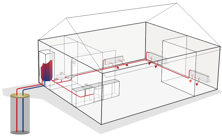
Тепловой коллектор скалистых пород
