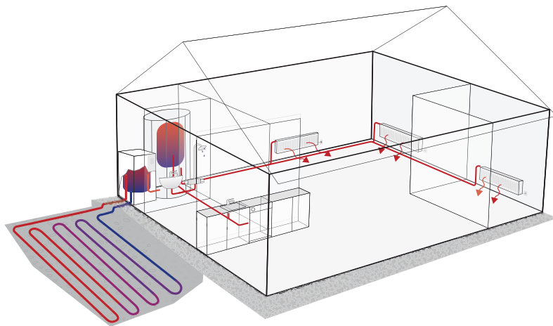
Тепловой контур коллектора геотермального насоса
