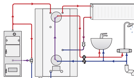
Твердотопливный котел YPV всегда подключается к аккумулятору энергии (например, Ovali).
