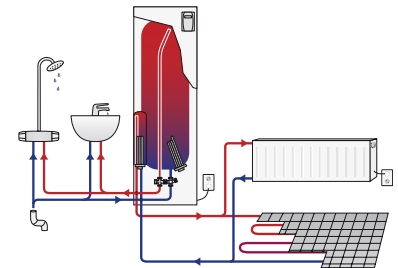
В Tehowatti объединены электродкотел и водонагреватель.
