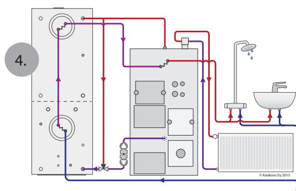
3. GTV Teknik с системой солнечных коллекторов 4. GTV Teknik с комбинированным котлом
