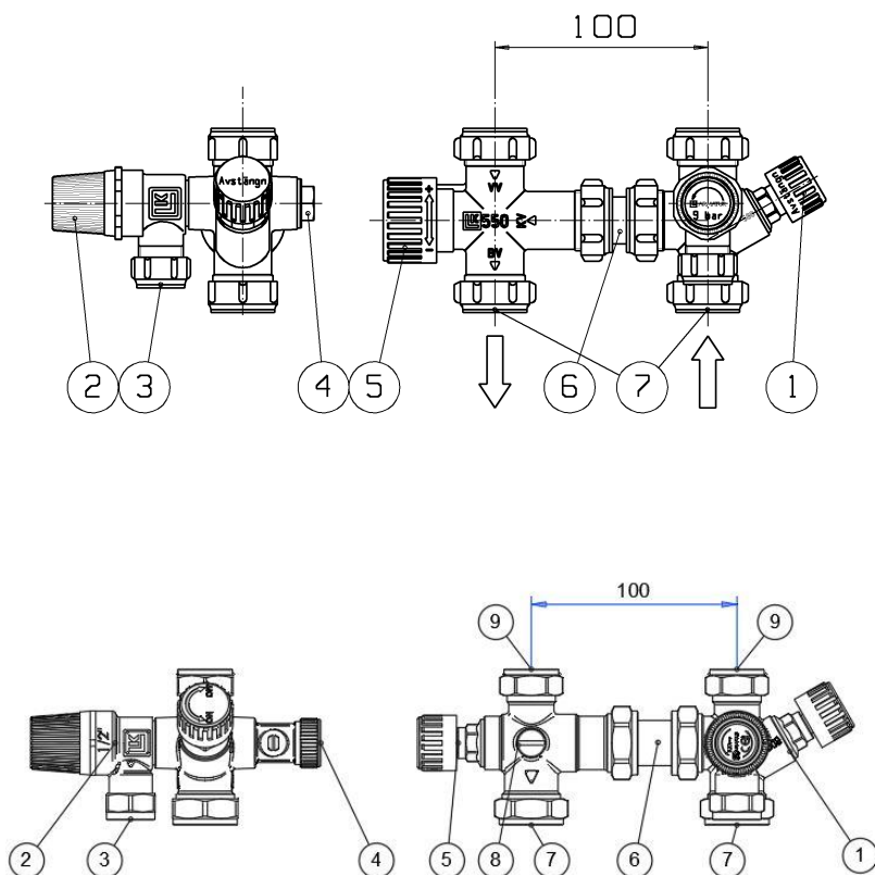
ЛК-КЛАПАННАЯ ГРУППА Ø 22/18*
