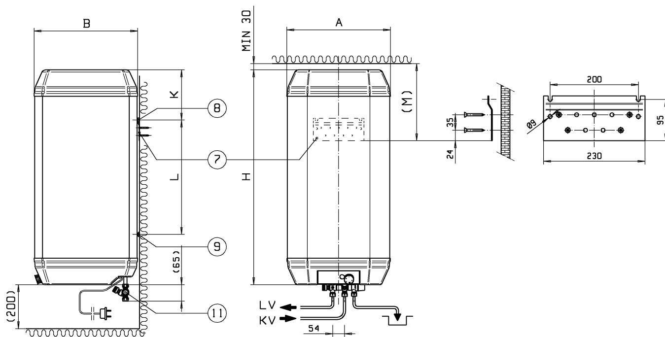
Рис. 2 Настенный монтаж водонагревателя Внимание! MIN 30 размер в модели VLK 160 составляет 50 мм.
