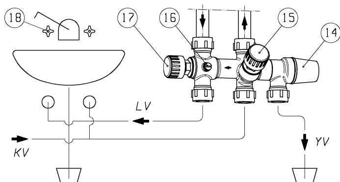
Рис. 8 Компоненты наполнения- / дренажа водонагревателя
